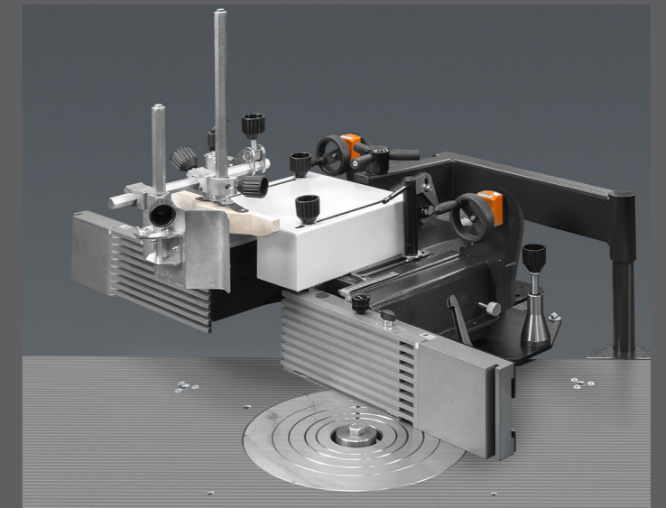
Machine met opties Machine avec options Maschine mit verschiedene Optionen Machine with several options
