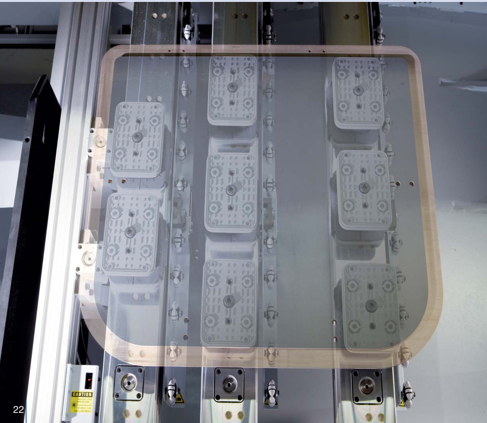
Konsolentisch für die exakte und flexible Teilefixierung
