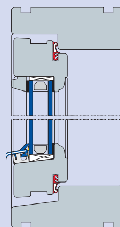
Fensterschnitt IV 116 nach außen öffnend
