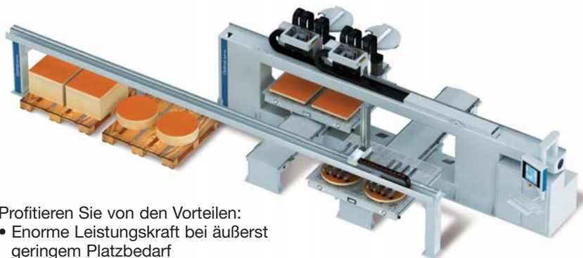
Beschicker TBP 370 in Synchronausführung für Linienportale der Baureihen B600 und B700
