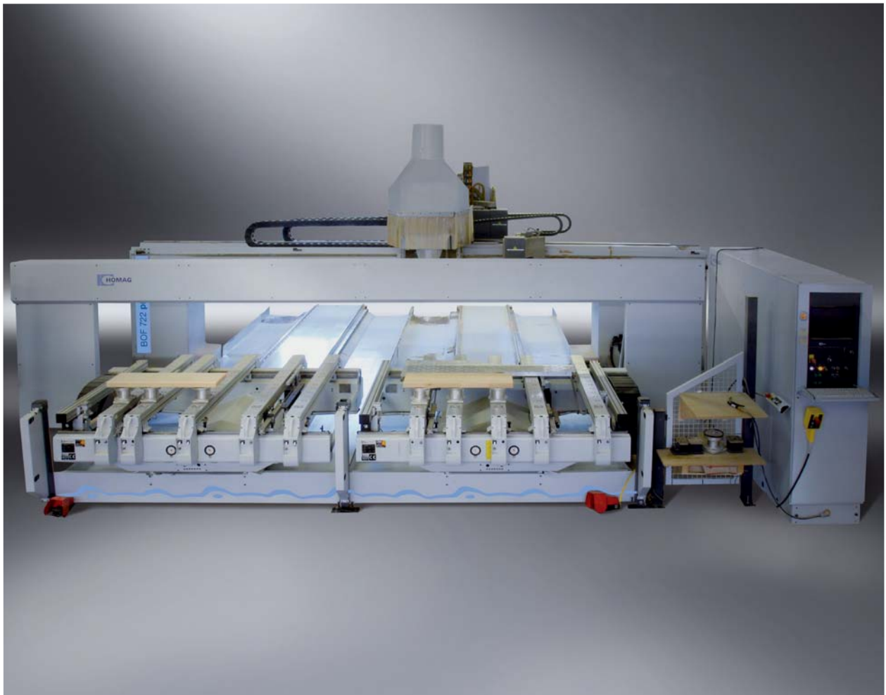
Bearbeitungszentren mit 5-Achs- und 4-Achs-Spindel zum zeitgleichen Bearbeiten von Handlaufkrümmungen und Treppenstufen
