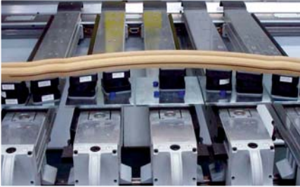
Durch das Maxi-Flex-Spannsystem entsteht eine durchgängige Ebene zur beliebigen Spannmittelpositionierung
