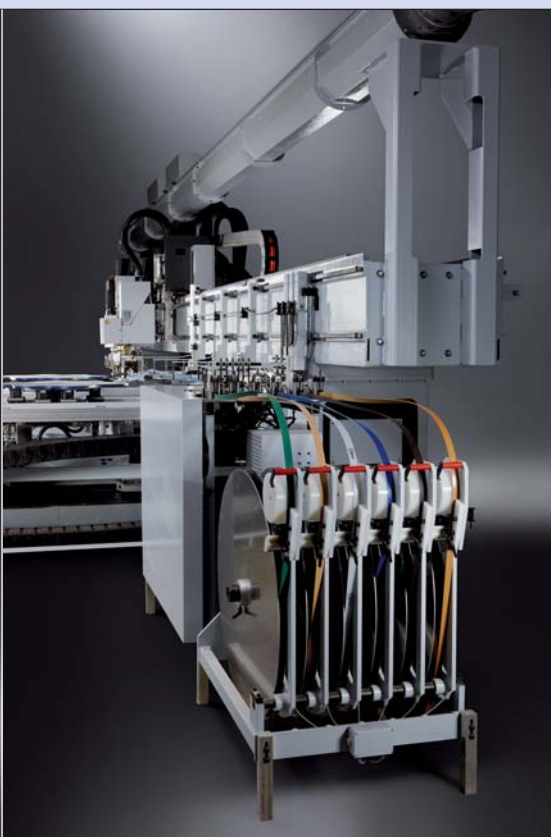
Kantenmagazin mitfahrend in X mit bis zu 6 Rollen oder extern mit bis zu 24 Rollen
