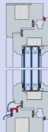
Fensterschnitt IV 101 für Passivhäuser
