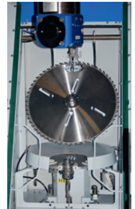
8-fach Werkzeugwechsler mit Pickup- Station
