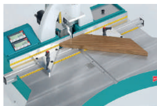
Frézování 45°
