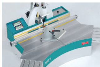
Pracovní stůl
