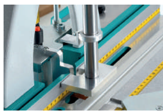
Nastavení výšky frézování a omezovač páky
